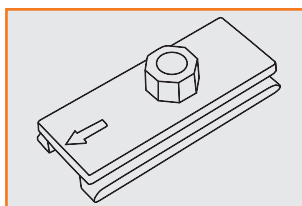
SHOP-NR. 10177 ITEM NO. 8206 Befestigungsplatte für breite Gabelbrücken Mounting plate for flat crown forks
